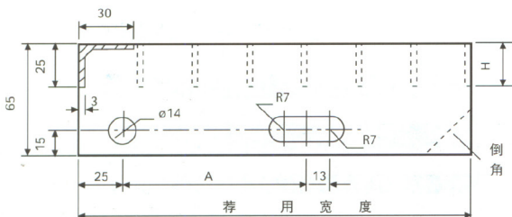
ST3 焊接固定，无花纹板，前护板
